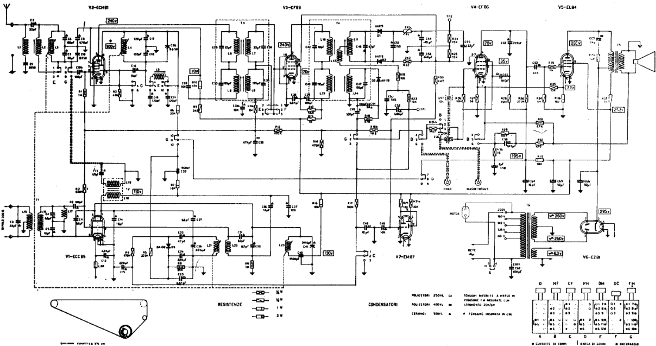
Schema elettrico del radiorecettore ULTRAVOX Mod. Explorer
